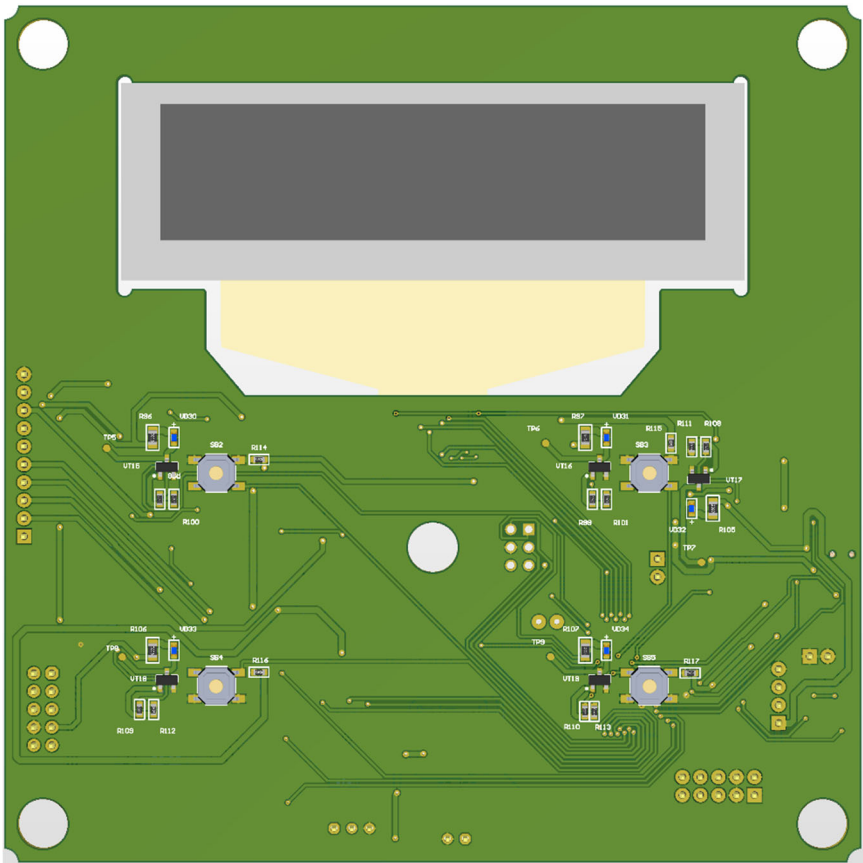
Рисунок 1. Печатная плата панели управления. Вид спереди.
