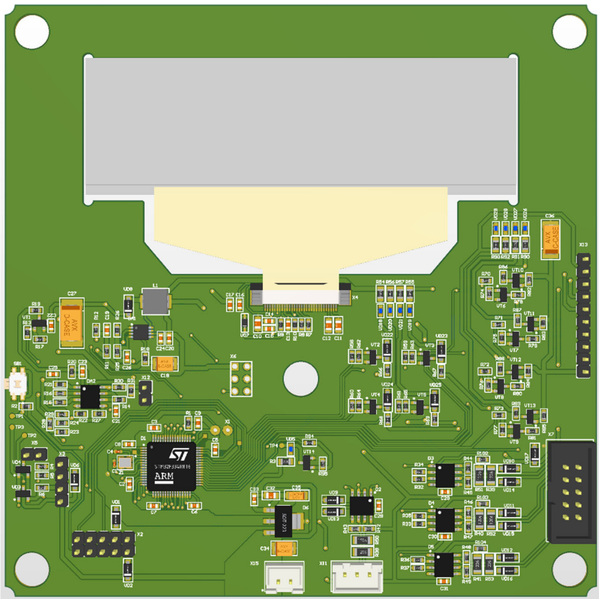
Рисунок 2. Печатная плата панели управления. Вид сзади.
